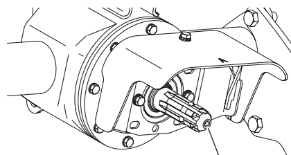
グリス塗布
