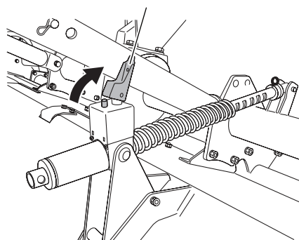
エプロンハネアゲロックレバー
