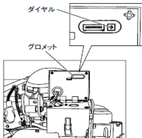
パッチングジョウ解除
