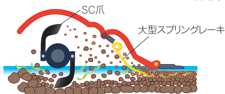
(スランディングカット爪) 特許番号 第3214248号
