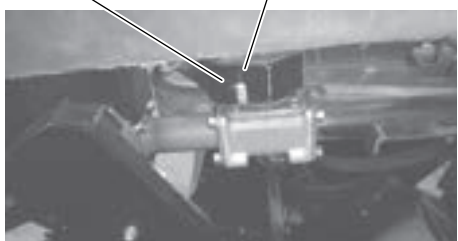
収穫部駆動 チェンカバー 注油口(左右 1 か所ずつ、 合計 2 か所)
