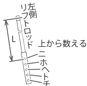
トップリンク・リフトロッド調整
