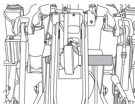
※拡大図
