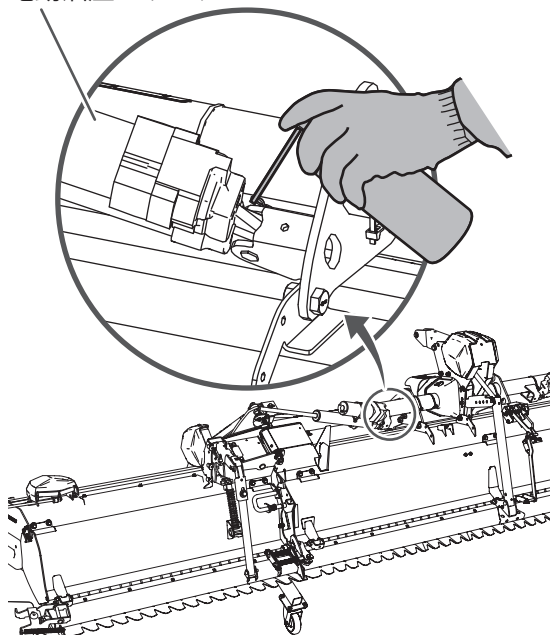
電動油圧シリンダ
